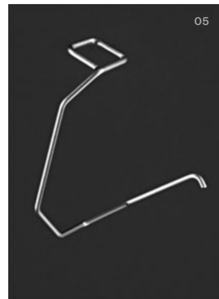
Haltefeder, rostfrei | d=1,3 mm
